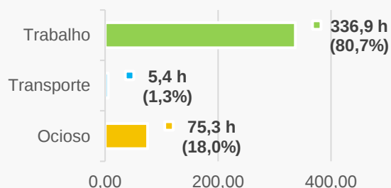
Tempo de uso da máquina (h)
