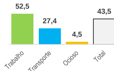
Consumo médio de combustível (L/h)
